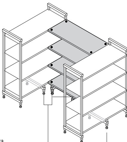
Unidad en forma de 'U' Dos unidades base + estantes intermedios
