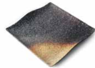
SQP2828-LAV 28 x 28 x 2,5 cm alto Uds. caja: 6
